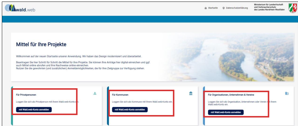
Abb. 1: Anmeldemaske Cockpit
